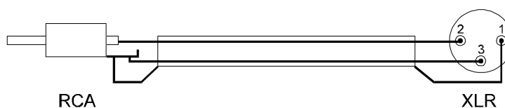
Obr. 2. Kábel pre nesymetrické prepojenie.
