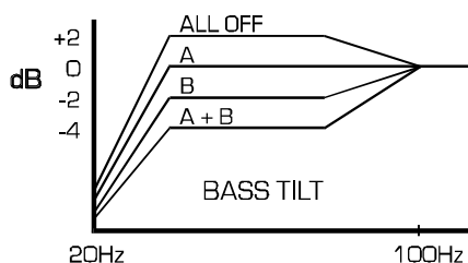
Obr. 8. Význam prepínačov „bass tilt“.
