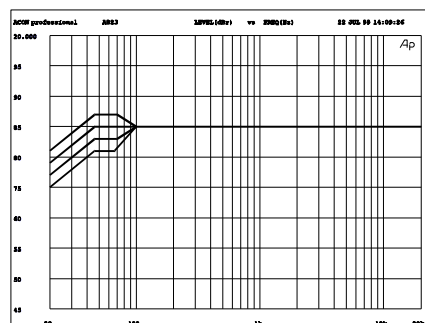
Obr. 7. Vplyv prepínača „bass tilt“ na frekv. charakteristiku (zjednodušené).
